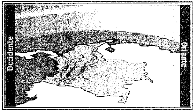
Posición actual aproximada del Sol respecto al país.
